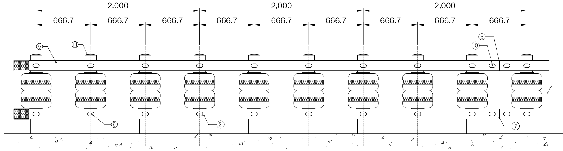
ELEVATION
