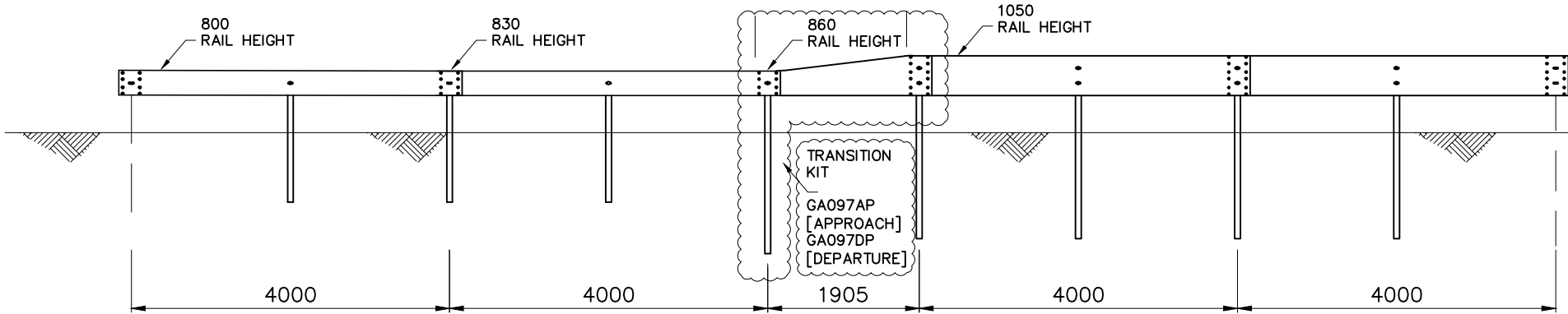
ELEVATION
